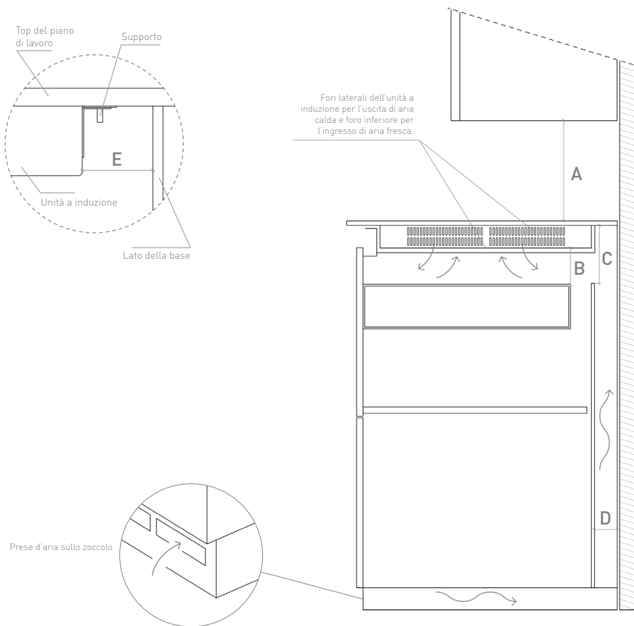
Fig 3: Distanze minime dalle basi e dai pensili della cucina Dettaglio dalla vista frontale
