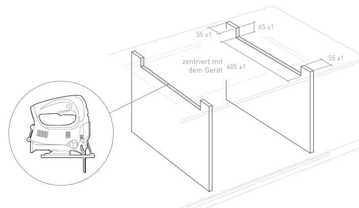
Abb. 2: Geben Sie die Seiten des Sockels form, wenn die empfohlenen Abstände in Abb. 3 nicht eingehalten werden können.
