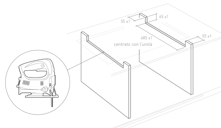
Fig 2: Sagomare i fianchi della base nel caso in cui non si possano mantenere le distanze raccomandate di Fig. 3.
