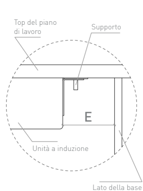
Fig 3: Distanze minime dalle basi e dai pensili della cucina Dettaglio dalla vista frontale
