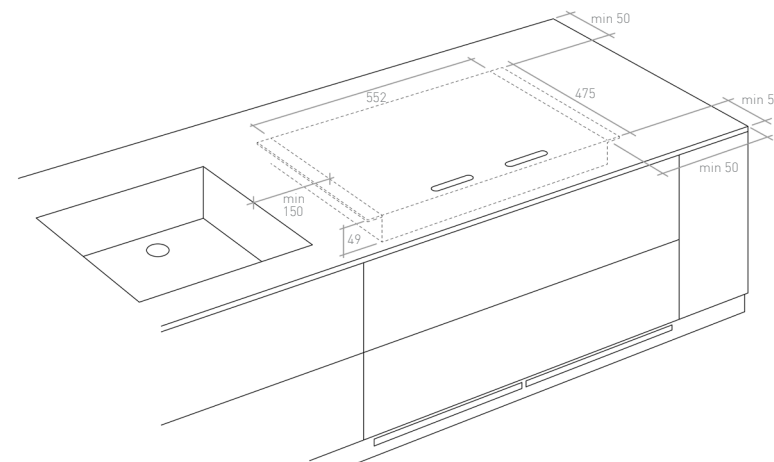
Fig 1: Dimensioni dell'unità a induzione e distanze minime dai bordi (50mm) e dai fori (150mm) del piano di lavoro.
