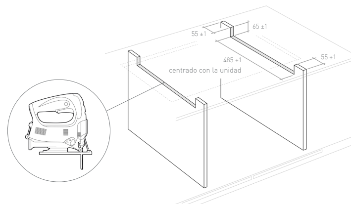
Fig 2: Modelar los laterales de la base si no se pueden mantener las distancias recomendadas en la Fig. 3.
