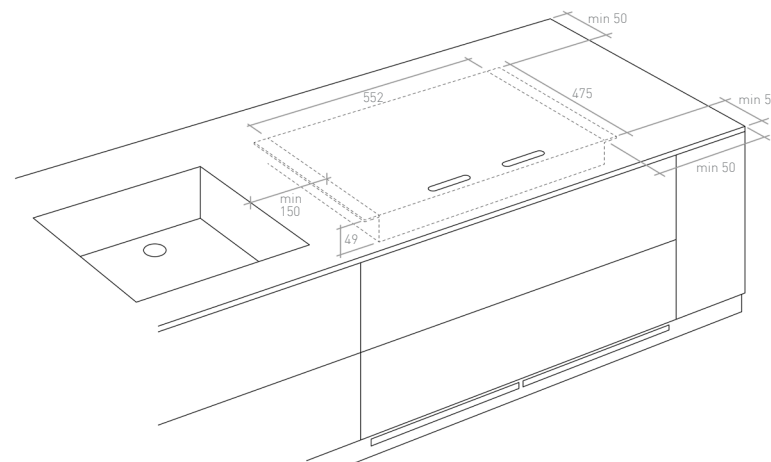
Fig 1: Dimensiones de la placa de inducción y distancias mínimas desde los bordes (50mm) y orificios (150mm) de la superficie de trabajo.
